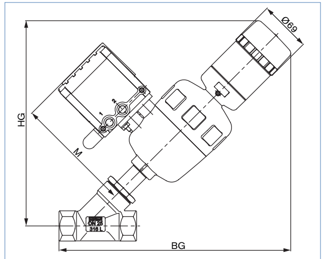
Система регулировки 2702 + 8635
